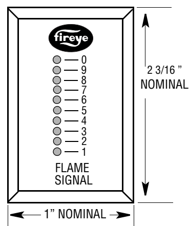
FACE DIMENSIONS
